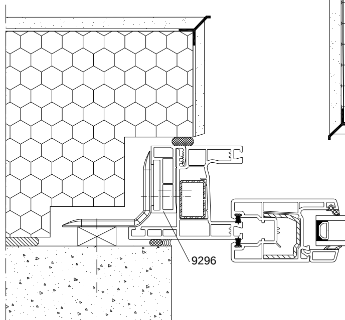
Coupe A-A
