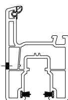
Drainage en façade
