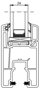
Double vitrage Vitrage isolant
