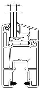
Simple vitrage RUP et PTOM uniquement
